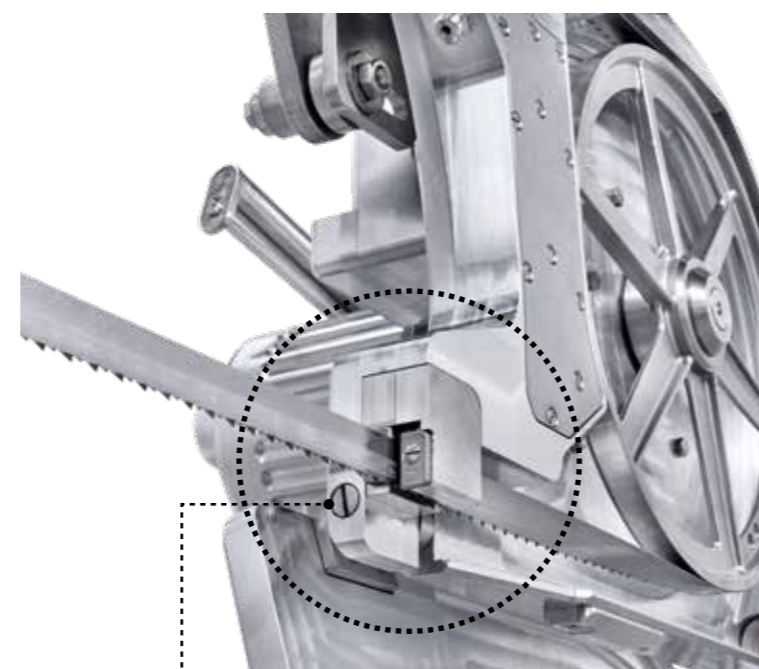
verbesserte Bandführung
