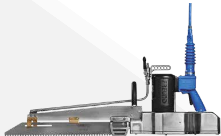
▶ SH60-03 - Spalt-Hubsäge
